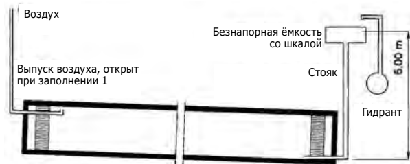
Рис. 10 Проверка герметичности
