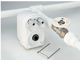
Фото 1. Шаровый кран, электропривод и скоба крепления
