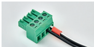
Фото 19. Подключение внешнего блока питания +12 В к ответной части разъема электропривода
