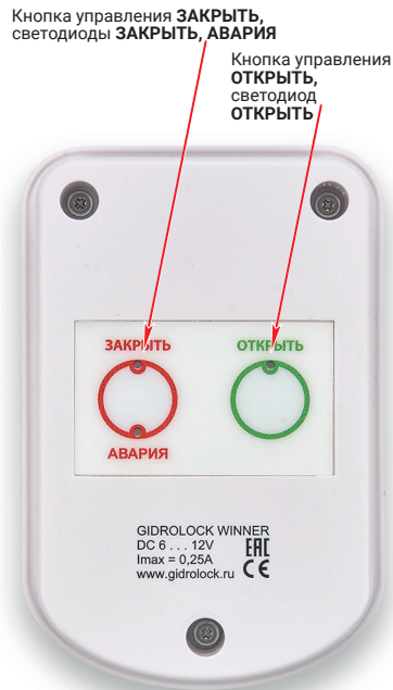
Фото 8. Элементы управления на корпусе шарового электропривода
