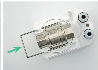
Фото 6. Крепление электропривода к шаровому крану с помощью металлической скобы
