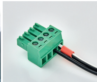
Фото 23. Подключение внешнего блока питания +12 В к ответной части разъема электропривода
