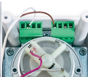
Фото 11. Подключение датчика к электроприводу
