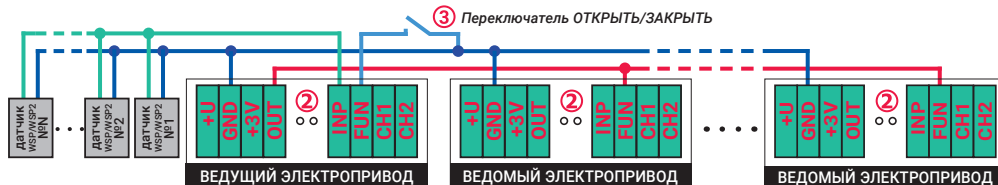
Рис. 2. Объединение в систему нескольких шаровых электроприводов из серий GIDROLOCK WINNER RADIO и GIDROLOCK WINNER
