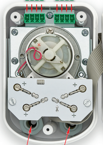
Фото 6. Электропривод управления шаровым краном со снятой крышкой
