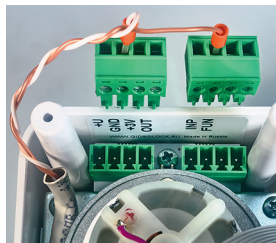
Фото 18. Подключение проводного выключателя к электроприводу
